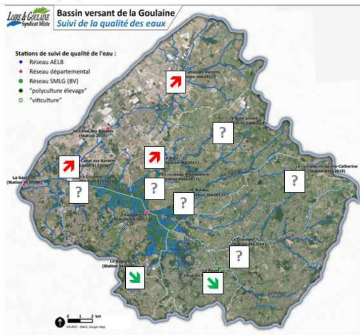
Figure 48: Evaluation qualité de l'eau sur le paramètre phytosanitaire
